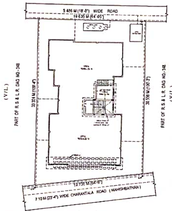
SITE PLAN SCALE - 1:1
